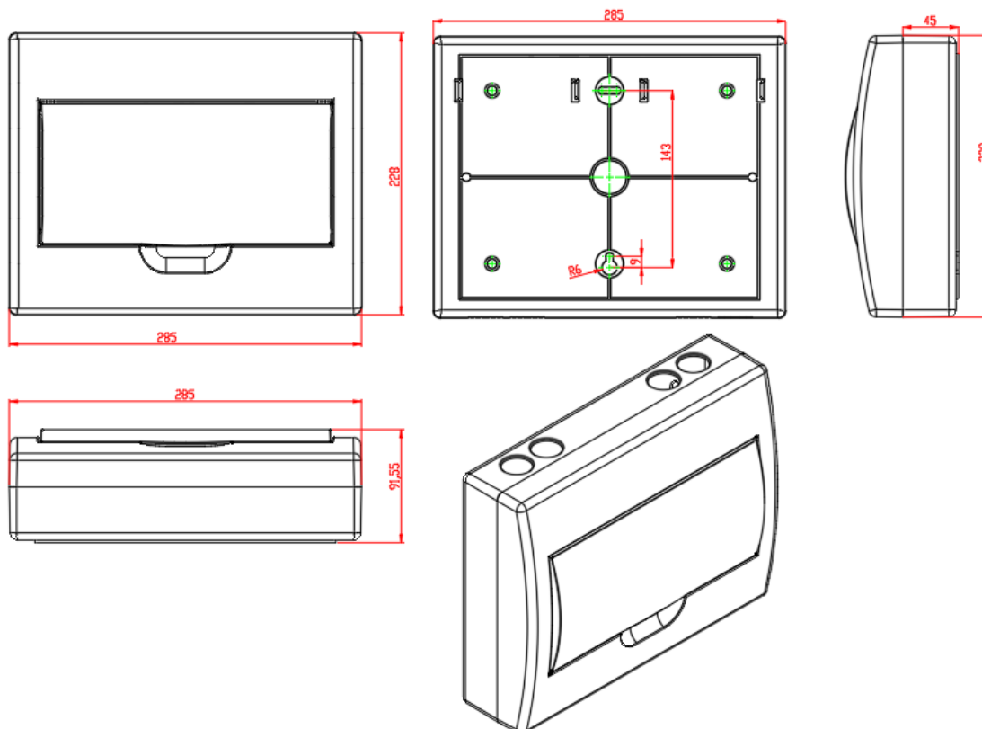
Figura 2.1: Dimensões do Gabinete Avalon (Cota em mm).
