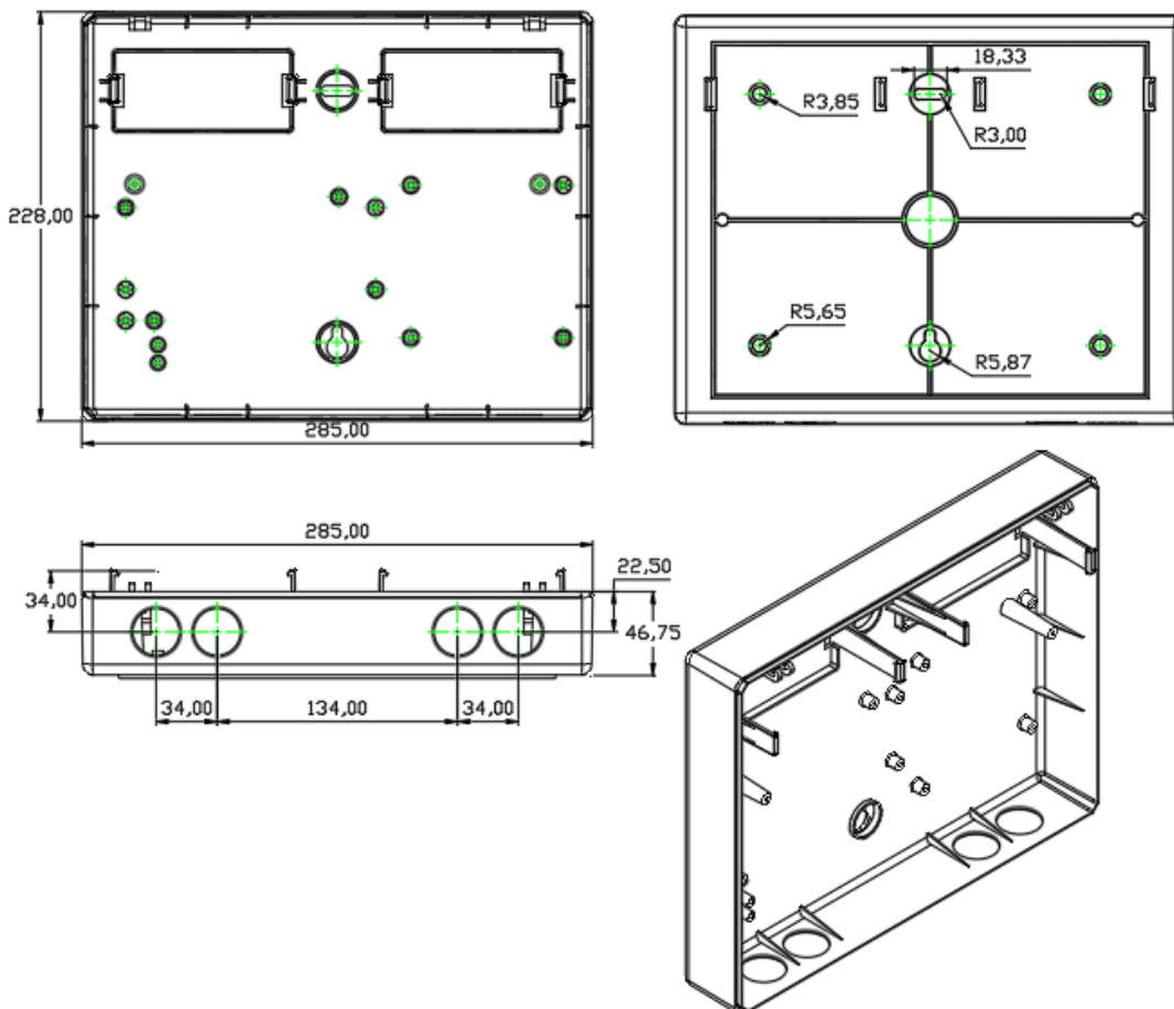
Figura 2.2: Fixação do Gabinete Avalon (Cota em mm).
